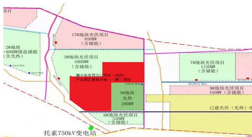
图 1.1 光伏场区地理位置示意图
